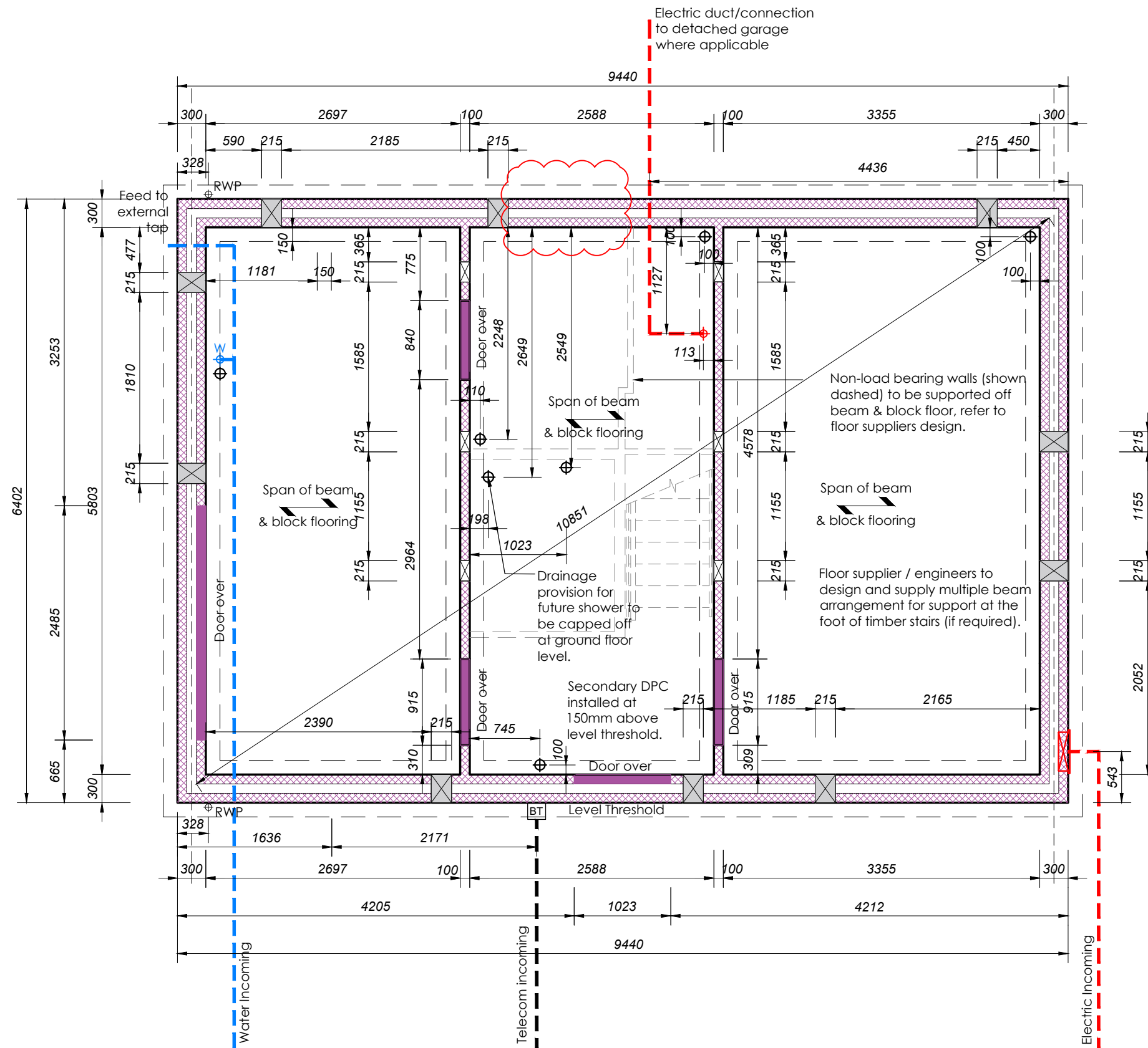
GOSFORD V2 (G02) - SUBSTRUCTURE PLAN Scale 1:50
