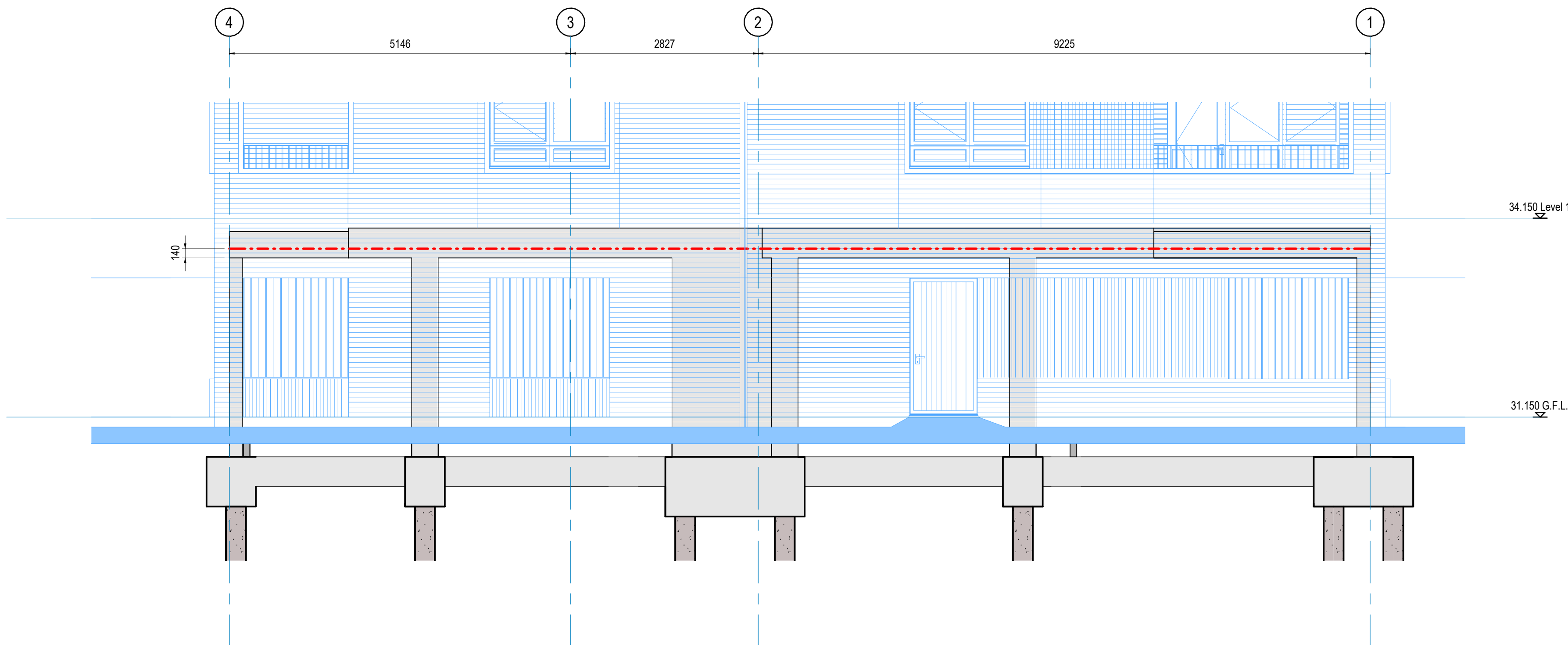
Elevation B (G.L. G / F) SCALE 1:50
