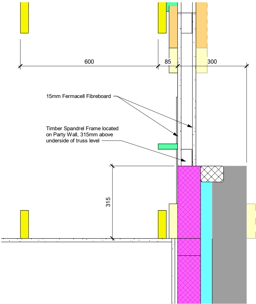
X Section X-X (Spandrel) 1 : 10
