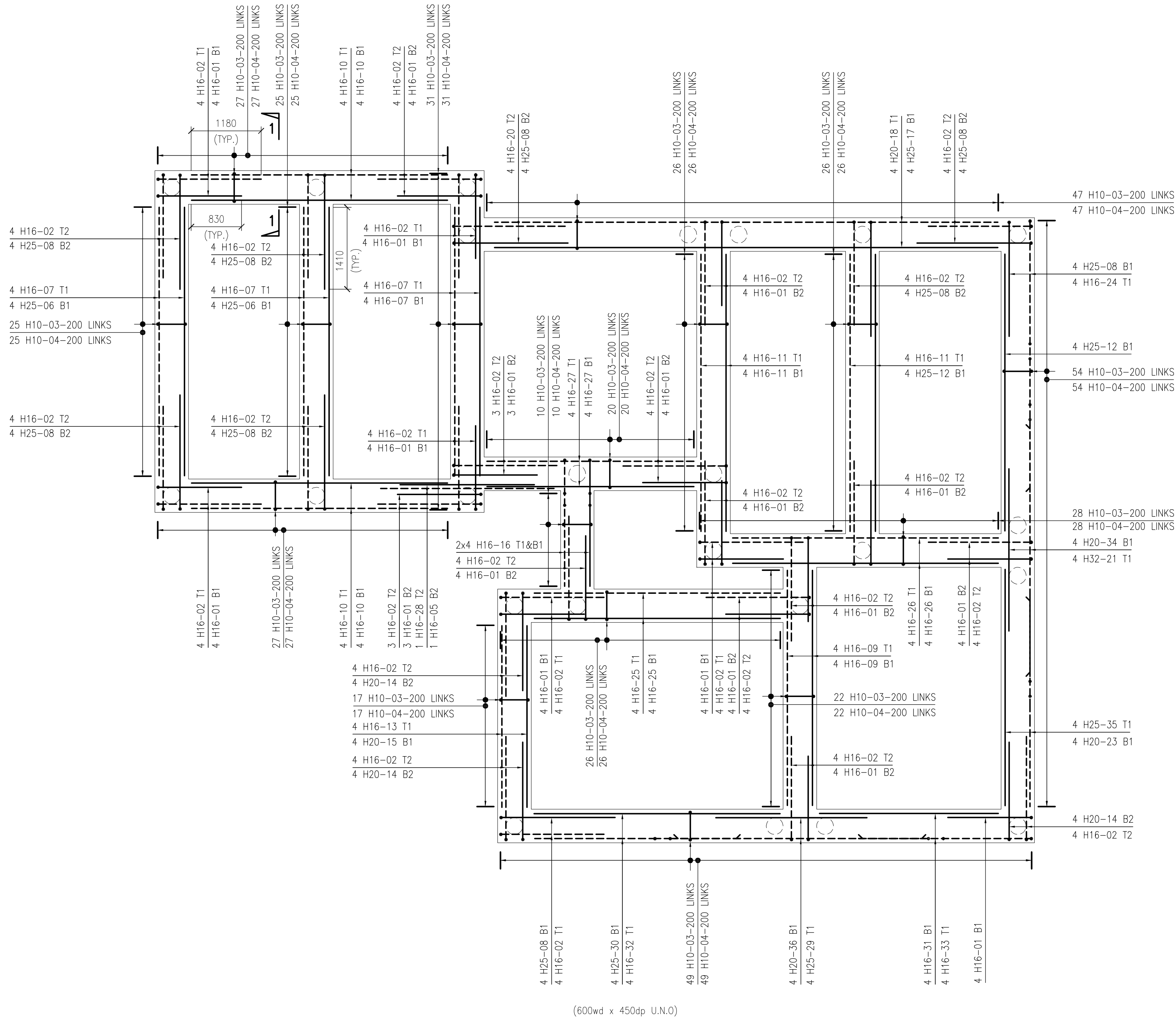
PLOT-652 'LEDHAM' SCALE 1:50
